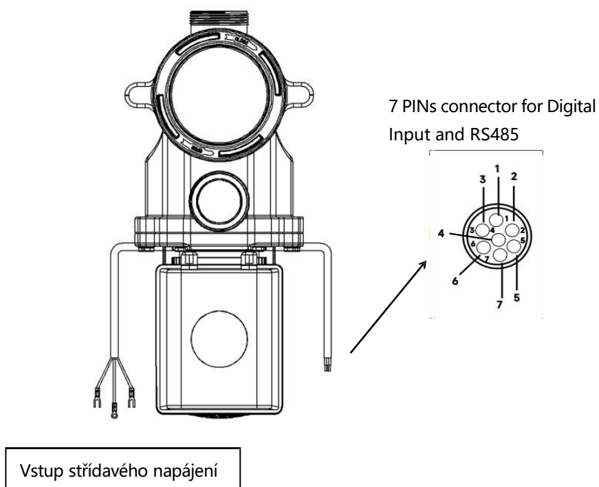
Obrázek 5 - Konektor digitálního vstupu
