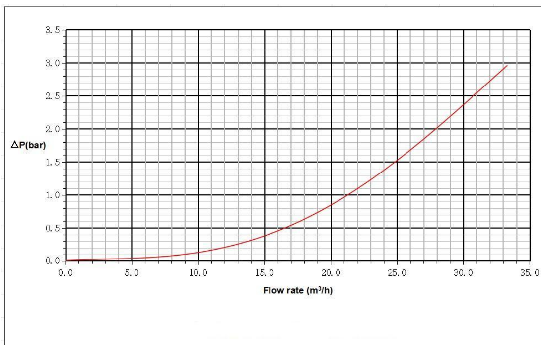
Obrázek 1 - Křivka tlakové ztráty - Filtrační režim
