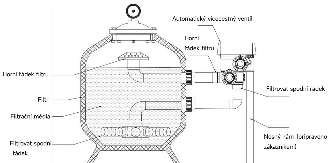
Obrázek 4 – Schéma instalace
